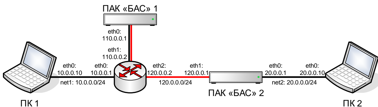
Рисунок 1 – Схема стенда
