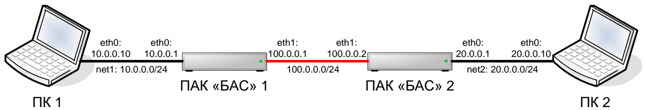
Рисунок 1 – Схема стенда
